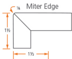
COUNTER EDGE
