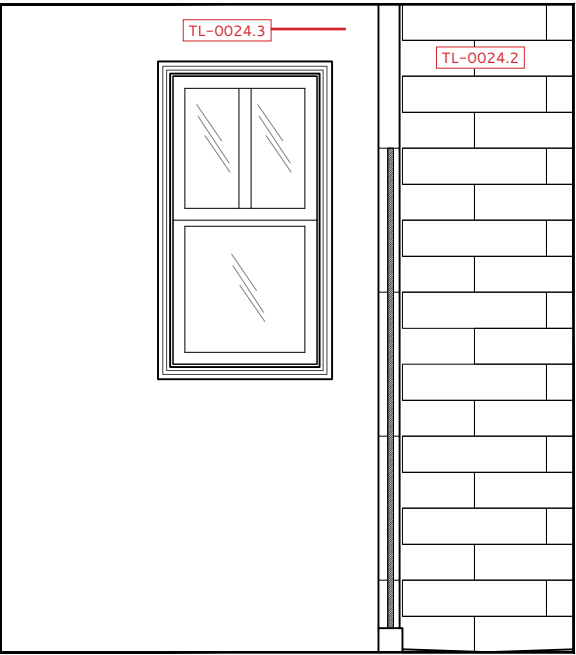
BATH 2 024 - ELEVATION B
