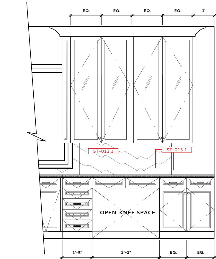
KITCHEN 013 - ELEVATION I SCALE: 3/8" = 1'-0"
