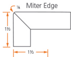
COUNTER EDGE
