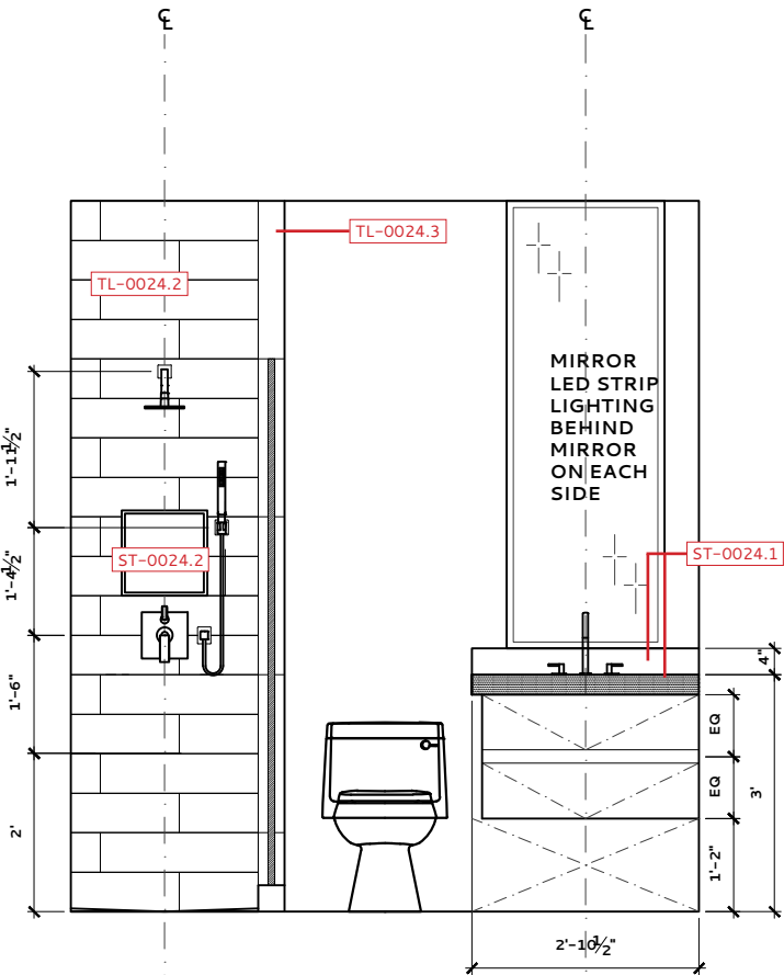
BATH 2 024 - ELEVATION D
