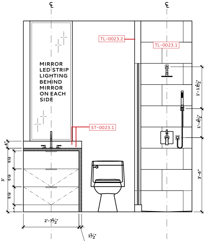
BATH 3 023 - ELEVATION D
