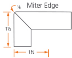
COUNTER EDGE
