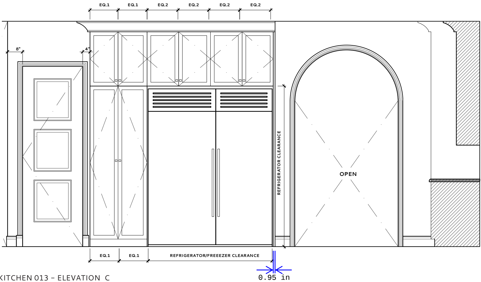
KITCHEN 013 - ELEVATION C SCALE: 3/8" = 1'-0"
