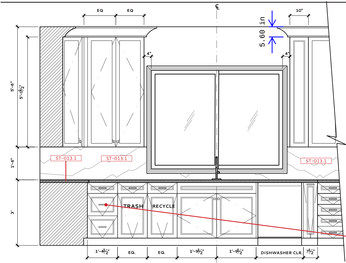
KITCHEN 013 - ELEVATION A SCALE: 3/8" = 1'-0"
